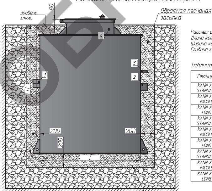
Монтажная схема станций KANN серии X
